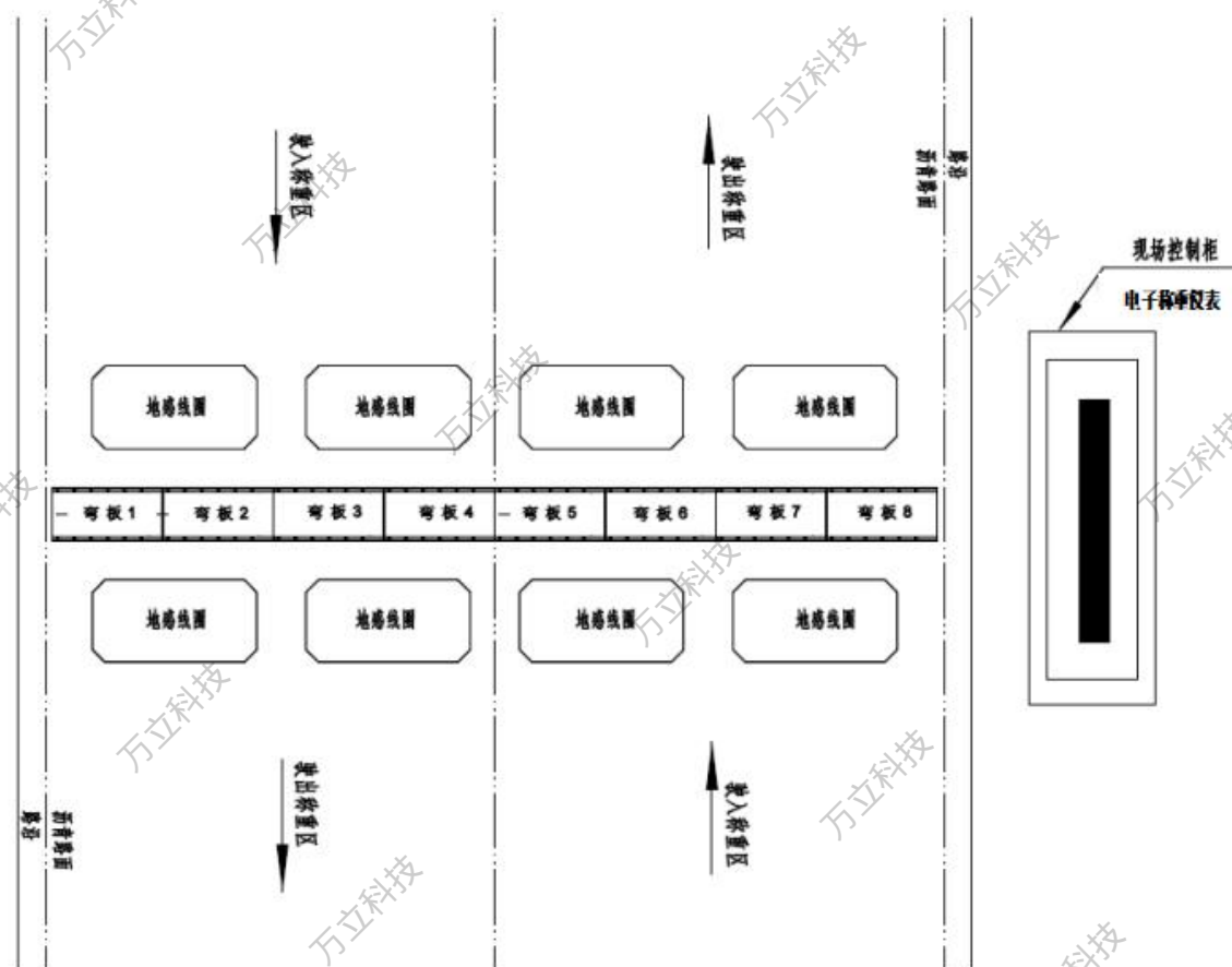
图 3-1 系统结构图
